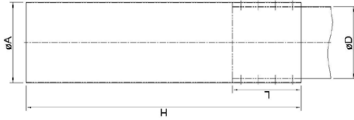
Detail Abschlagrohr
