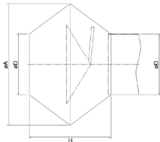
Detail Deflektorkopf
