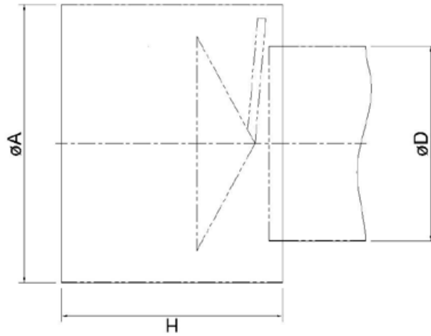
Detail Deflektorkopf
